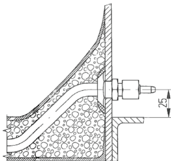
Anschluss Saugleitung
