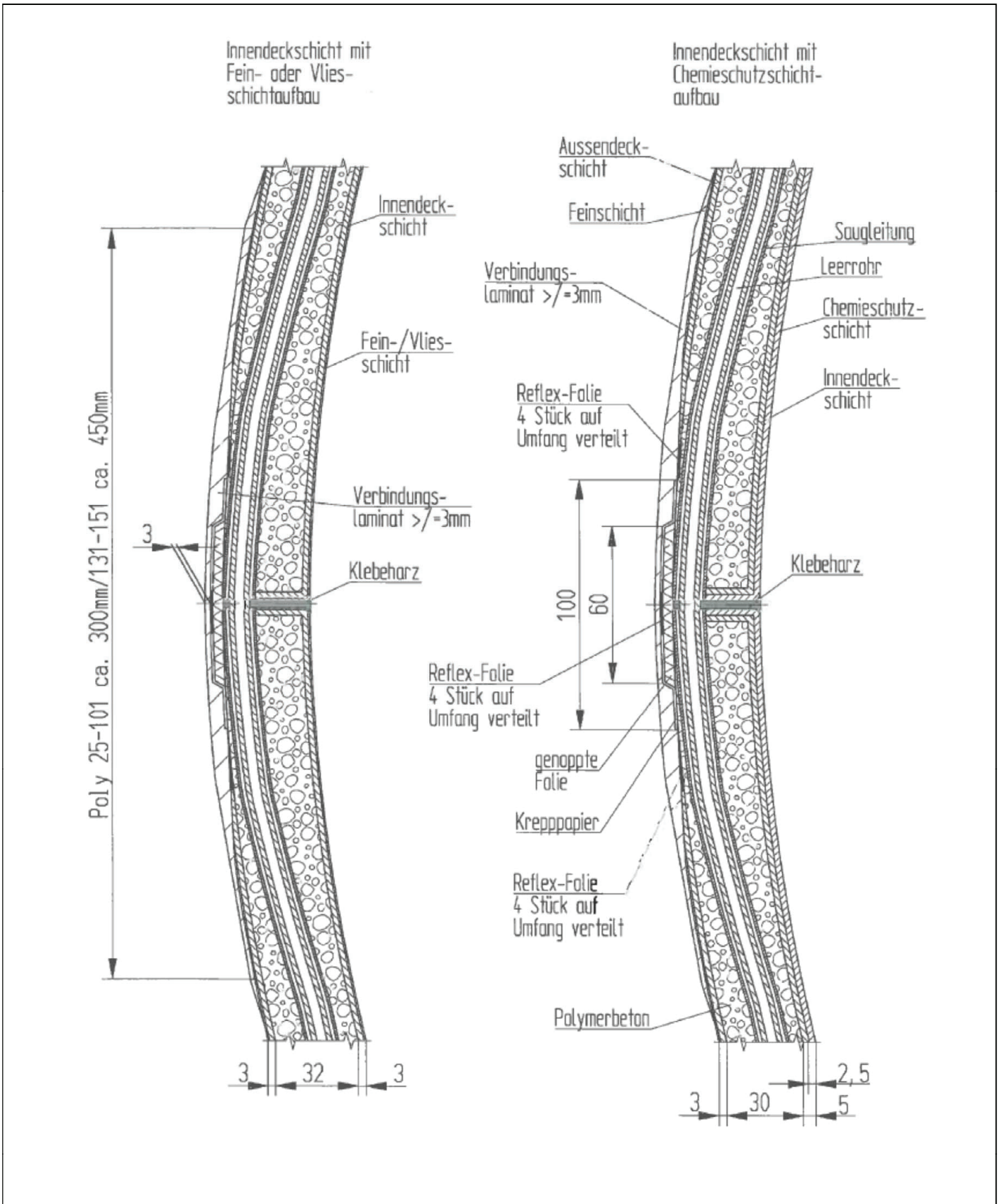
Mehrschichtige kugelhähnliche Behälter Poly 25/35/51/61/81/101/131/151
